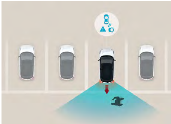
Asystent zapobiegania kolizjom z pieszymi podczas jazdy do tyłu (PCA-R) Ciesz się dodatkowym bezpieczeństwem podczas manewrowania w wąskich miejscach parkingowych na wstecznym biegu. W przypadku wykrycia ryzyka kolizji z pieszym lub przeszkodą system ostrzega i automatycznie włącza hamulce.
