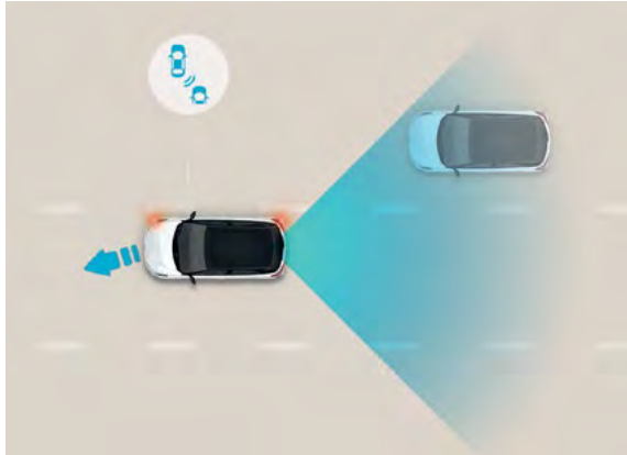
Aktywny system monitorowania martwego pola (BCA) Korzystając z dwóch czujników radarowych w dolnym tylnym zderzaku, system ostrzega o pojazdach poruszających się w martwym polu. Jeśli włączysz kierunkowskaz, system uaktywni alarm dźwiękowy, a następnie zahamuje, aby uniknąć przewidywanej kolizji.
